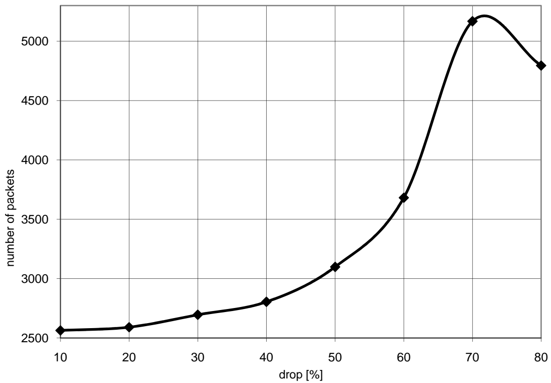
Diagramm fifa_drop2: Fifa 2007 drop 2
