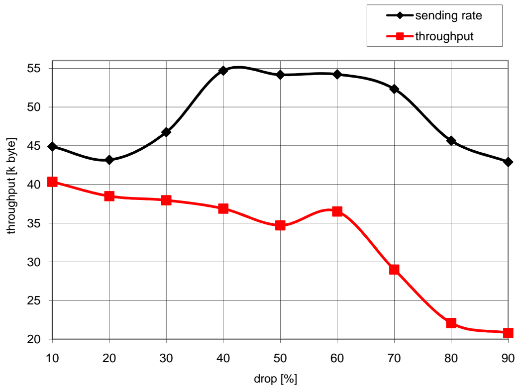
Diagramm dow_drop3: Dawn of War drop 3
