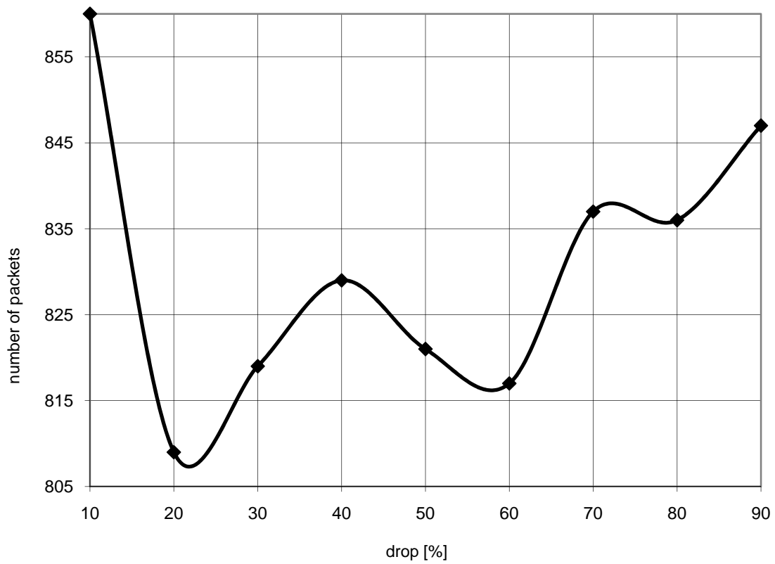
Diagramm dow_drop2: Dawn of War drop 2
