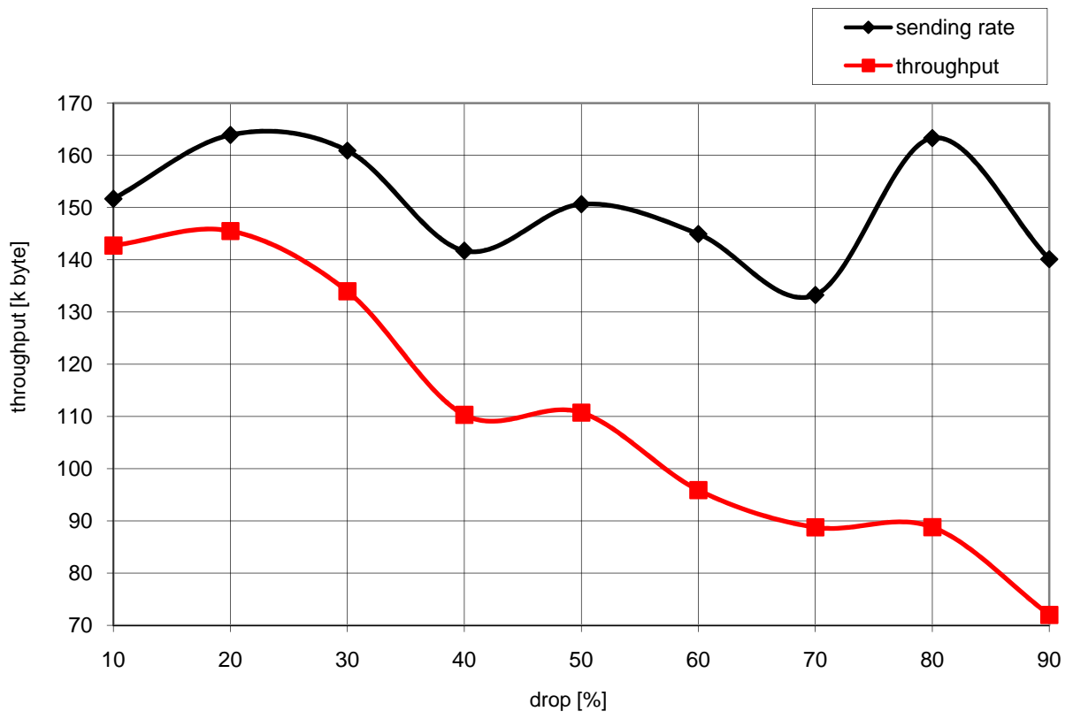
Diagramm q4_drop3: Quake 4 drop 3
