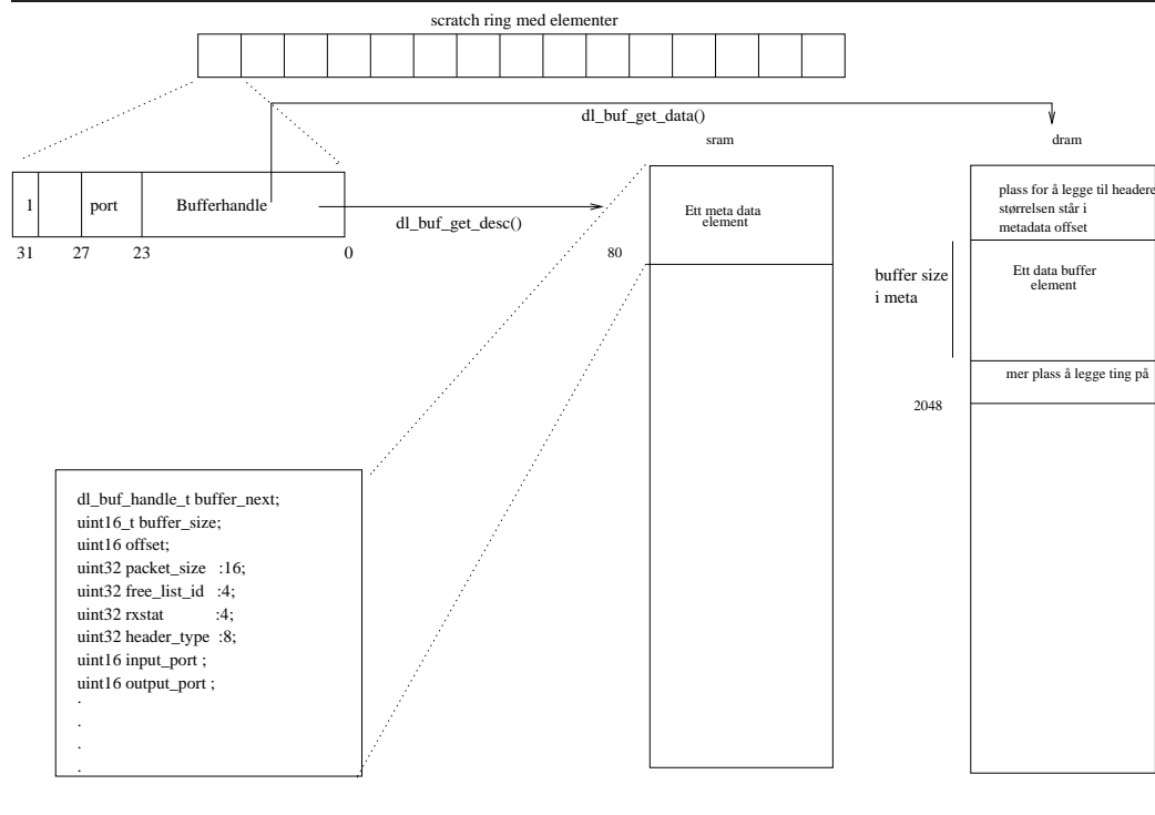
Figur 3.4 Bufferdeskriptor
